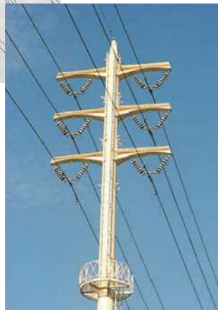
送電線は高い電圧の電気を流しておりますので、電線を支える支持物は、主に鉄塔が使われています。
